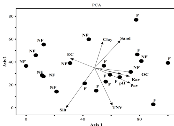
شکل ۵- رجن بندی خصوصیات فیزیکی و شیمیایی خاک مورد بررسی در فضای دو مؤلفه اول و دوم (EC: هدایت الکتریکی، Clay: درصد رس، Sand: درصد شن، OC: کربن آلی، Kav: پتاسیم در دسترس، pH: اسیدیته، TNV: آهنک و Silt: درصد سیلت)
