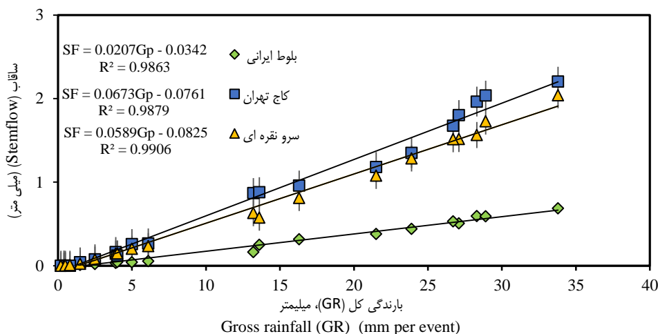
شکل ۴- نمودار بین بارندگی در هر بارش (GR) و ساقاب (SF) و برازش خط لگاریتمی برای سه توده Figure 4. Scatterplot for rainfall (mm) and stemflow (mm) and logarithmic fit pooled for three studied stands
