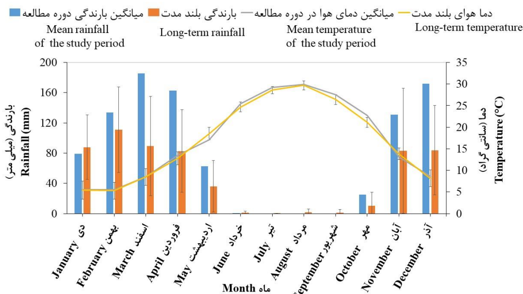
شکل ۲- میانگین درجه حرارت و بارندگی ماهیانه بر اساس آمار سی و چهار ساله (از سال ۱۳۶۵ تا سال ۱۳۹۹) ایستگاه سینوپتیک شهر ایلام (نزدیک‌ترین ایستگاه هواشناسی به منطقه مورد مطالعه) Figure 2. Monthly mean rainfall and air temperature based the past 34 years (1986-2020), as recorded by a nearby synoptic meteorological station (approximately 500 m away)
