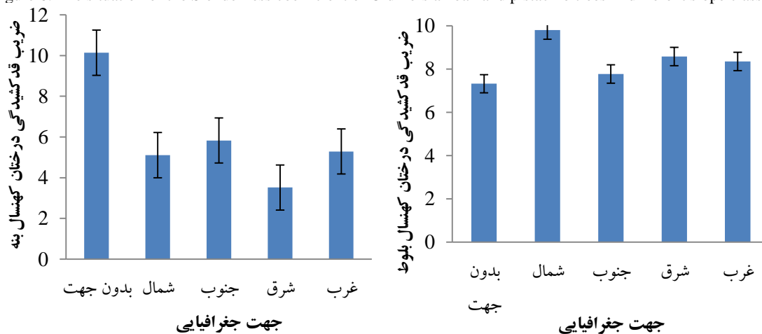
شکل ۷- وضعیت ضریب قد کشیدگی درختان کهنسال بلوط ایرانی و بنه در جهت‌های جغرافیایی مختلف Figure 7. Status of the Slenderness coefficient of old Persian oak and pistachio trees in different aspects
