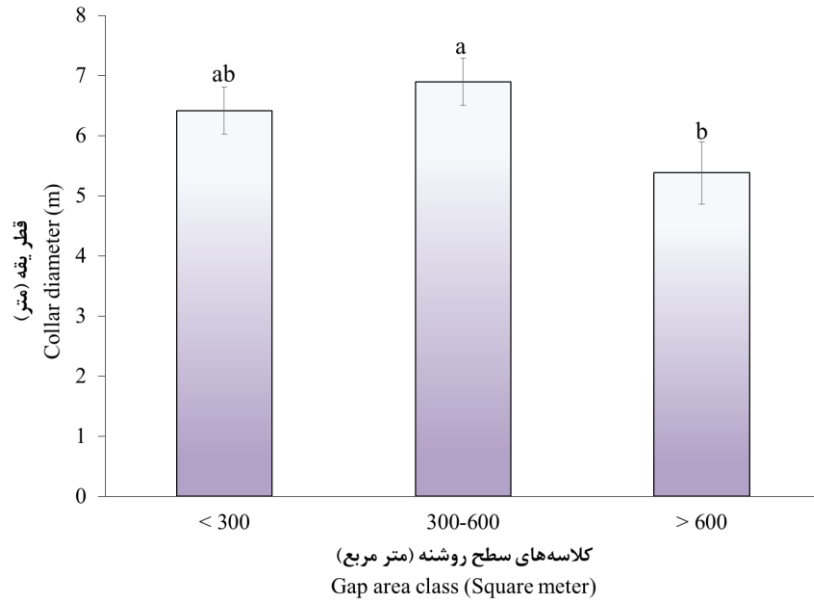
شکل ۱۱- مقایسه میانگین قطر یقه (سانتی‌متر) در کلاسه‌های مساحت روشنه (سطح معنی‌داری ۰/۰۵)
