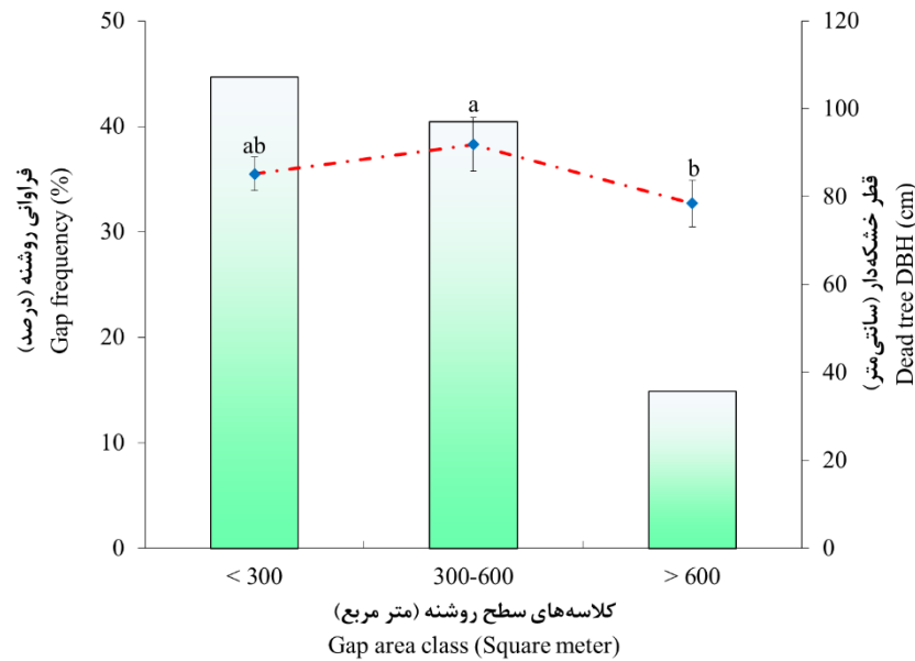
شکل ۲- فراوانی (درصد) روشنیه‌ها و میانگین قطر خشک‌دار در کلاسه‌های سطح روشنیه (سطح معنی‌داری ۰/۰۵) Figure 2. Frequency (percentage) of the gaps and mean diameter of dead trees in different gap area classes (0.05 significance level)
