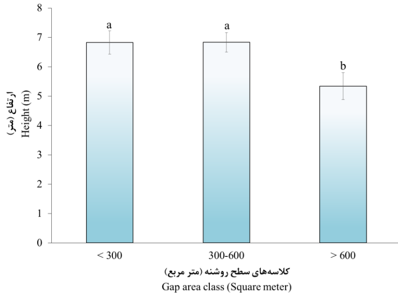
شکل ۱۲- مقایسه میانگین ارتفاع (متر) در کلاسه‌های مساحت روشنه (سطح معنی‌داری ۰/۰۵)
