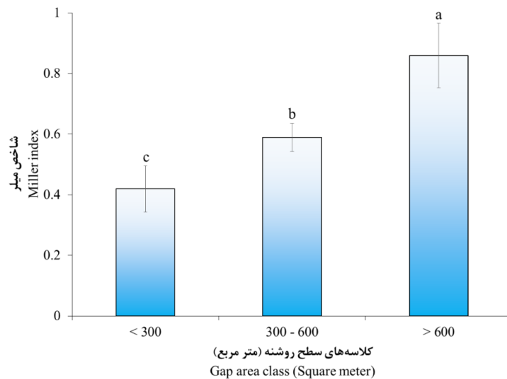
شکل ۵- مقایسه مقادیر شاخص کشیدگی میلر در کلاسه‌های سطح روشن (سطح معنی‌داری ۰/۰۵) Figure 5. Compares the miller elongation index values in the gap area classes (0.05 significance level)
