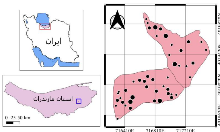
شکل ۱- منطقه مورد مطالعه در استان مازندران، ایران (دایره‌های مشکی نشان‌دهنده پراکندگی روشنه‌ها به صورت شماتیک است) Figure 1. Study area in Mazandaran province, Iran (The black circles indicate the schematic scatter of the gaps)
