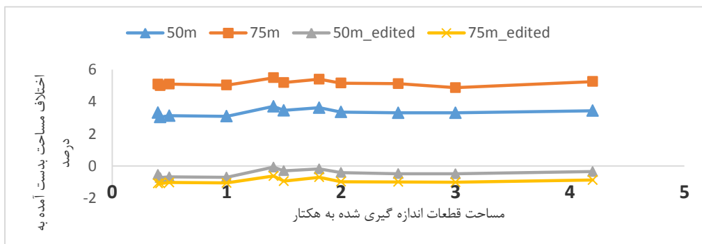
شکل ۱۴- نمودار اختلاف مساحی پهپاد نسبت تئودولیت بر حسب درصد پیش و پس از اعمال ضریب تصحیح Figure 14. UAV surveying difference diagram rather than GPS in percent before and after correction factor
