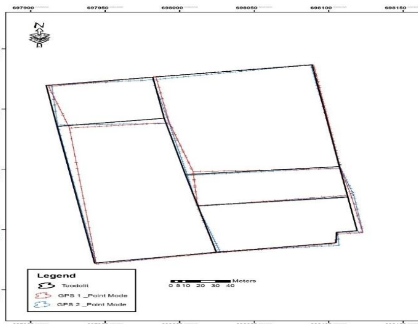
شکل ۲- نقشه تهیه شده با استفاده از GPS به روش برداشت نقطه و مقایسه آن با نقشه تهیه شده با تئودولیت Figure 2. Map prepared using GPS in point method and comparing with the map prepared with Teodolite
