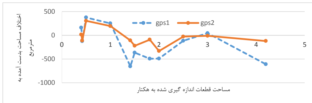
شکل ۳- نمودار اختلاف مساحتی GPS به روش برداشت نقطه نسبت به تئودولیت بر حسب مترمربع Figure 3. GPS surveying difference diagram in point method rather than Teodolite in square meter
