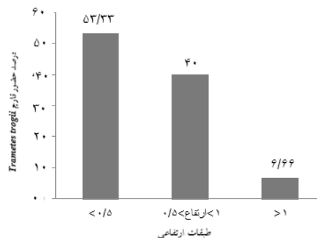
شکل ۱۲- بررسی درصد فراوانی قارچ Trametes trogii (Berk.) Dom در سه طبقه <۰/۵، ۱<ارتفاع<۰/۵ و >۱ متر Figure 12. The presence percentage of Trametes trogii (Berk.) Dom in three classes: <0.5, 1> height 0.5 and 1<
