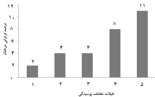
شکل ۱۳- درصد فراوانی درختان در طبقات مختلف پوسیدگی Figure 13. Percentage of trees in different decay classes
