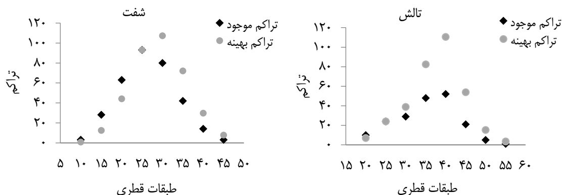
ادامه شکل ۳- منحنی‌های ابر نقاط مقادیر واقعی و بهینه تراکم در طبقات قطری در هر منطقه Continued Figure 3. Current and optimal density at DBH classes in each stand
