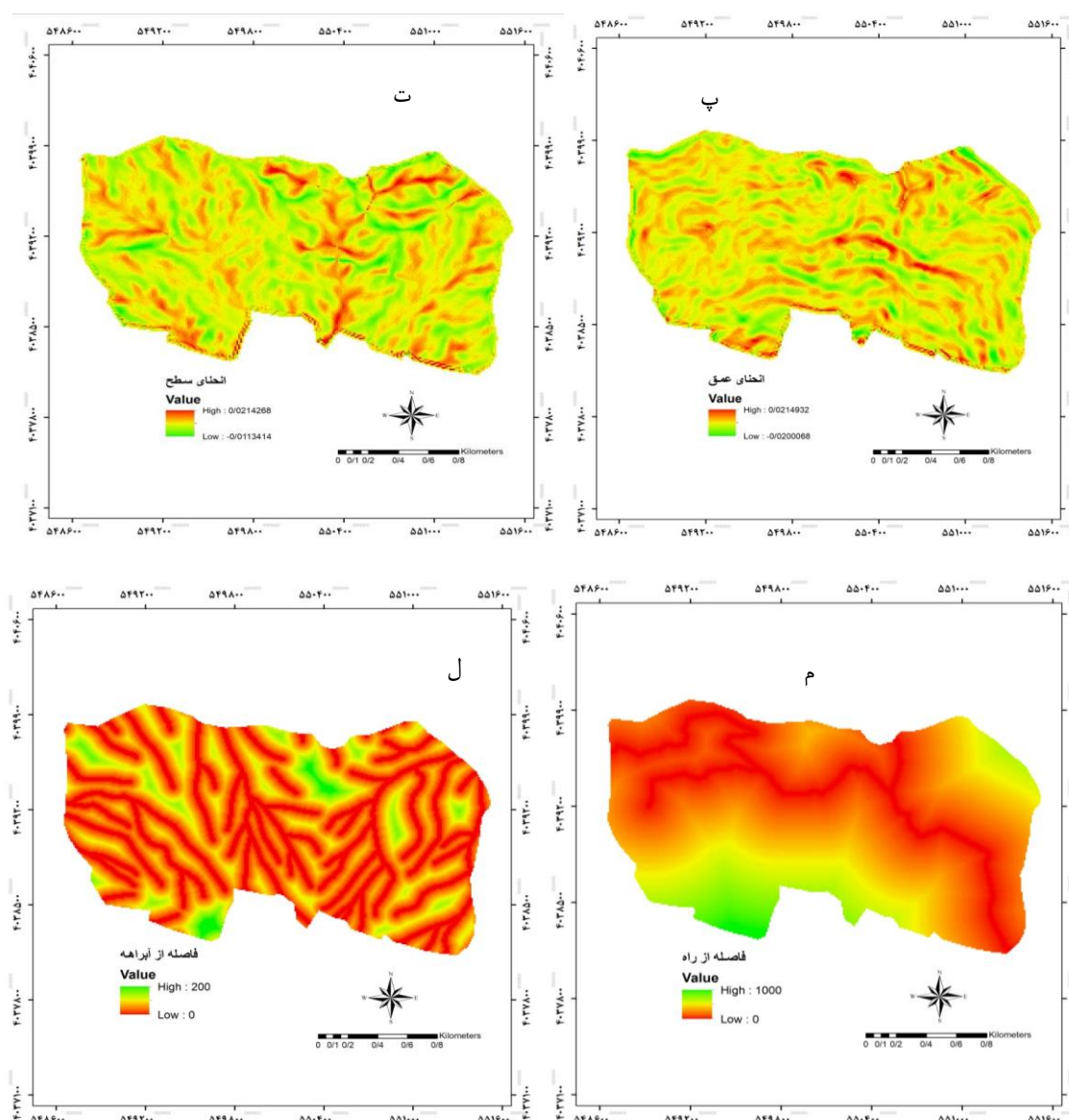
ادامه شکل ۲- نقشه عوامل مورد استفاده در این مطالعه شامل ارتفاع (الف)، جهت (ب)، شیب (ج)، شاخص خیس (د)، انحنای قائم (پ)، انحنای افقی (ت)، فاصله از آب‌راه (ل) و فاصله از راه (م).
