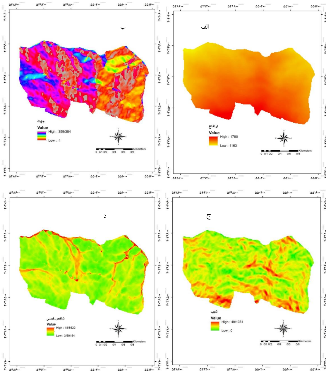
شکل ۲- نقشه عوامل مورد استفاده در این مطالعه شامل ارتفاع (الف)، جهت (ب)، شیب (ج)، شاخص خیس (د)، انحنای قائم (پ)، انحنای افقی (ت)، فاصله از آبراهه (ل) و فاصله از راه (م)
