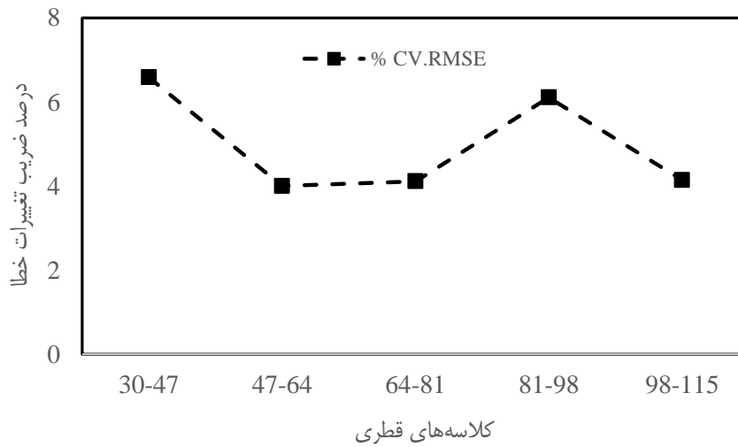
شکل ۵- مقدار درصد ضریب تغییرات خطا در کلاس‌های قطری مختلف قطر برابر سینه Figure 5. Value of % CV.RMSE in different diameter classes of diameter at breast height
