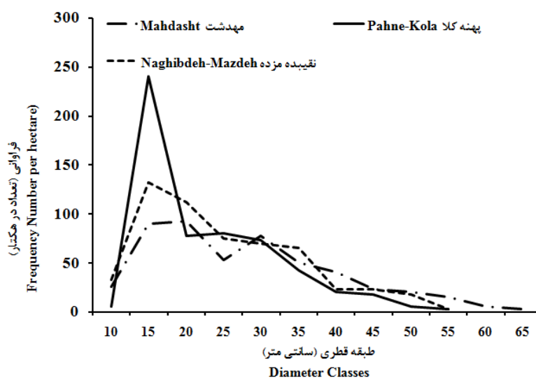
شکل ۲- پراکنش تعداد در طبقات قطری درختان صنوبر دلتوئیدس در رویشگاه‌های مختلف مورد مطالعه Figure 2. Distribution of Number of Populus deltoides trees per hectare in diameter classes in study sites
