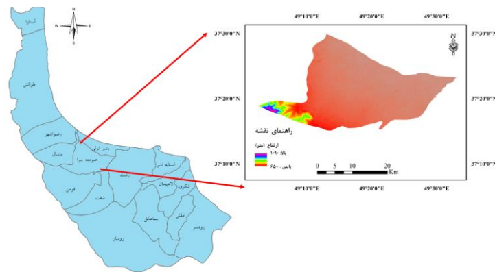
شکل ۱- موقعیت منطقه مورد مطالعه در استان گیلان Figure 1. Location of the study area in Gilan province
