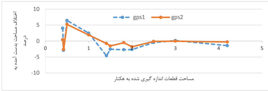
شکل ۴- نمودار میزان اختلاف مساحی GPS به روش برداشت نقطه نسبت به مساحی تئودولیت بر حسب درصد Figure 4. GPS surveying difference diagram in point method rather than Teodolite in percent
