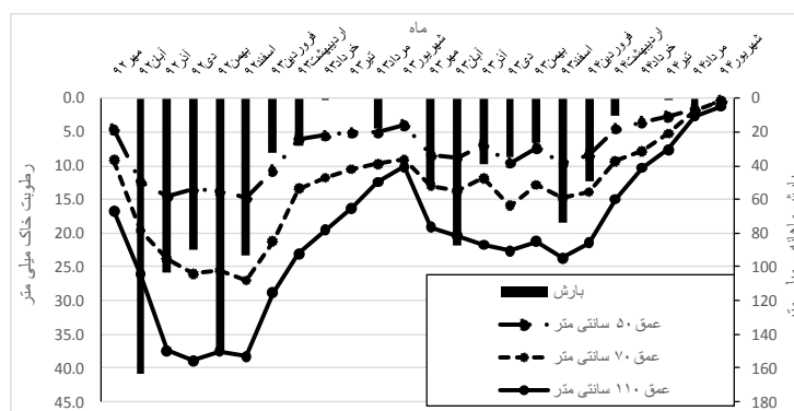
شکل ۲- تغییرات رطوبت خاک در عمق‌های ۵۰، ۷۰ و ۱۱۰ سانتی‌متری خاک در طی دوره بررسی در رویشگاه مله سیاه ایلام Figure 2. Changes in soil moisture at depths of 50, 70 and 110 cm during the period of review on the Melheh Siah Ilam
