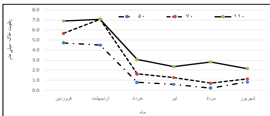
شکل ۳- نرخ کاهش ماهانه رطوبت خاک مربوط به دوره خشک سال در عمق‌های مورد بررسی در سال ۹۲-۹۳ در رویشگاه مله سیاه ایلام Figure 3. Monthly decreases in soil moisture related to the dry period at the depths studied in the year 2013-2014 on the habitat of Melheh Siah Ilam
