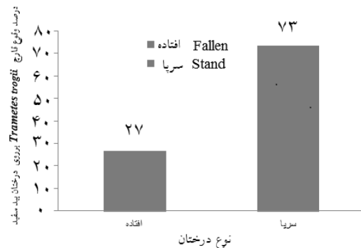
شکل ۸- درصد فراوانی قارچ Trametes trogii (Berk.) Dom روی درختان بید سفید
