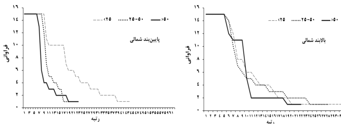
شکل ۶- نمودار رتبه - فراوانی تنوع گیاهی برای پوشش علفی در بالابند- دامنه شمالی (سمت راست) و پایین‌بند - دامنه شمالی (سمت چپ) Figure 6. Species abundance - ranking curve of herbaceous species in high land- north aspect (right) and low land- north aspect (left)
