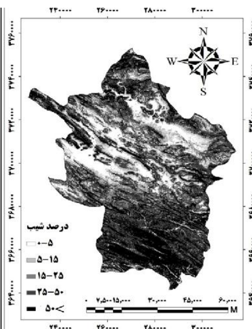
شکل ۳- نقشه شیب منطقه مورد مطالعه
