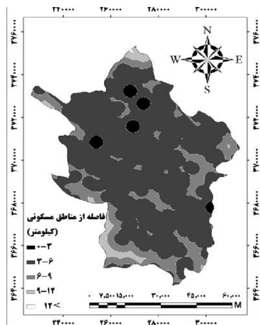
شکل ۱۲- نقشه فاصله از مناطق مسکونی منطقه مورد مطالعه
