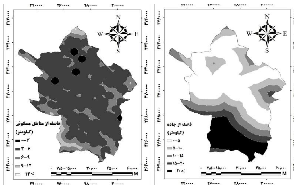
شکل ۱۱- نقشه فاصله از جاده‌های منطقه مورد مطالعه
