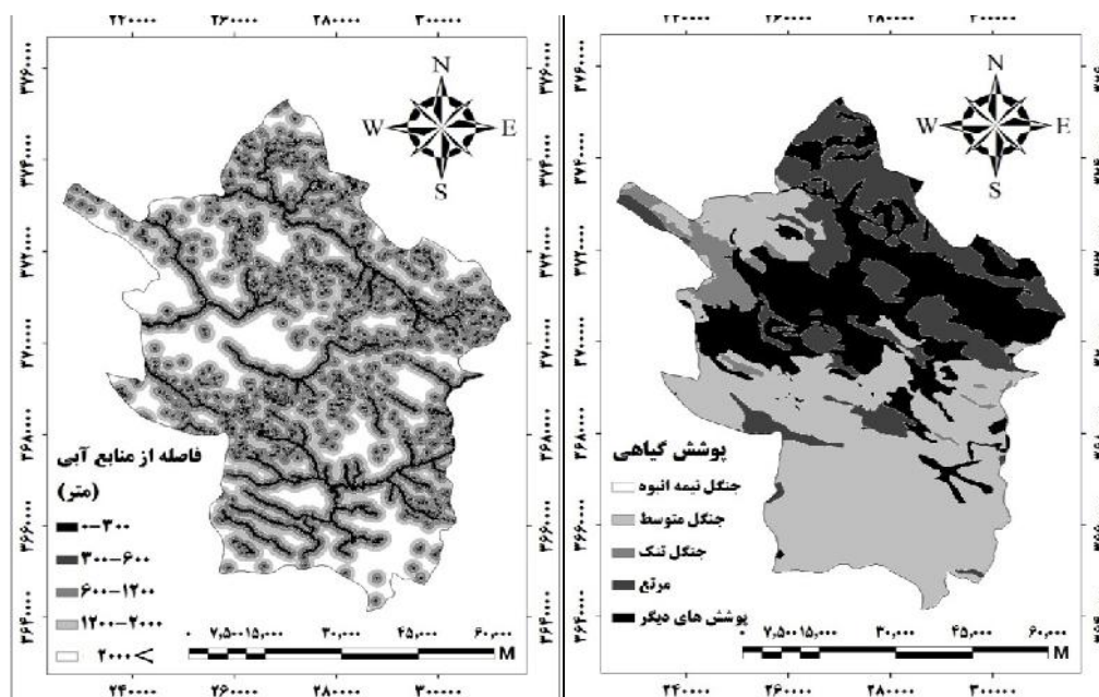
شکل ۹- نقشه پوشش گیاهی منطقه مورد مطالعه
