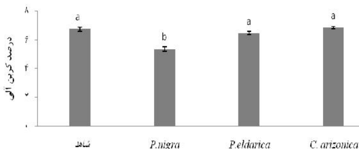
شکل ۲- مقایسه میانگین درصد کربن آلی در خاک‌های سوزنی‌برگان با شاهد
