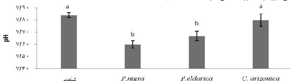
شکل ۱- مقایسه میانگین pH در خاک های سوزنی برگان با شاهد
