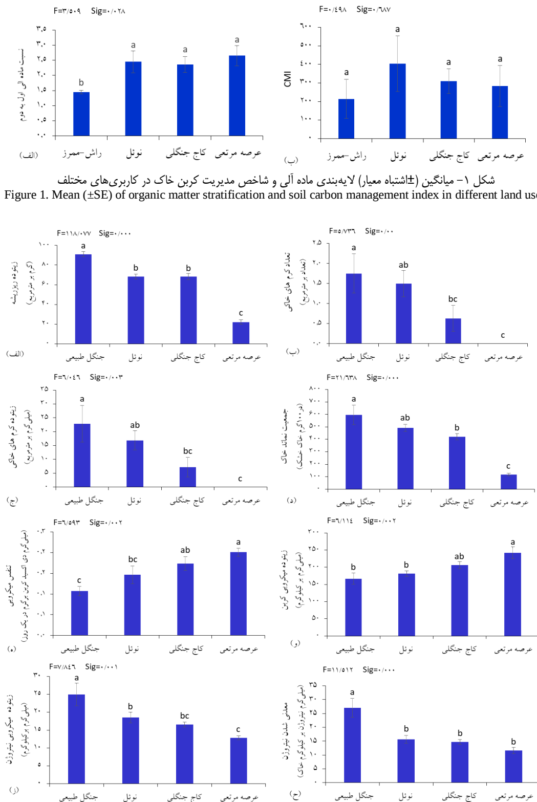
شکل ۲- میانگین (±اشتباه معیار) فعالیت‌های زیستی خاک در کاربری‌های مختلف Figure 2. Mean (±SE) of soil biological activities in different land uses
