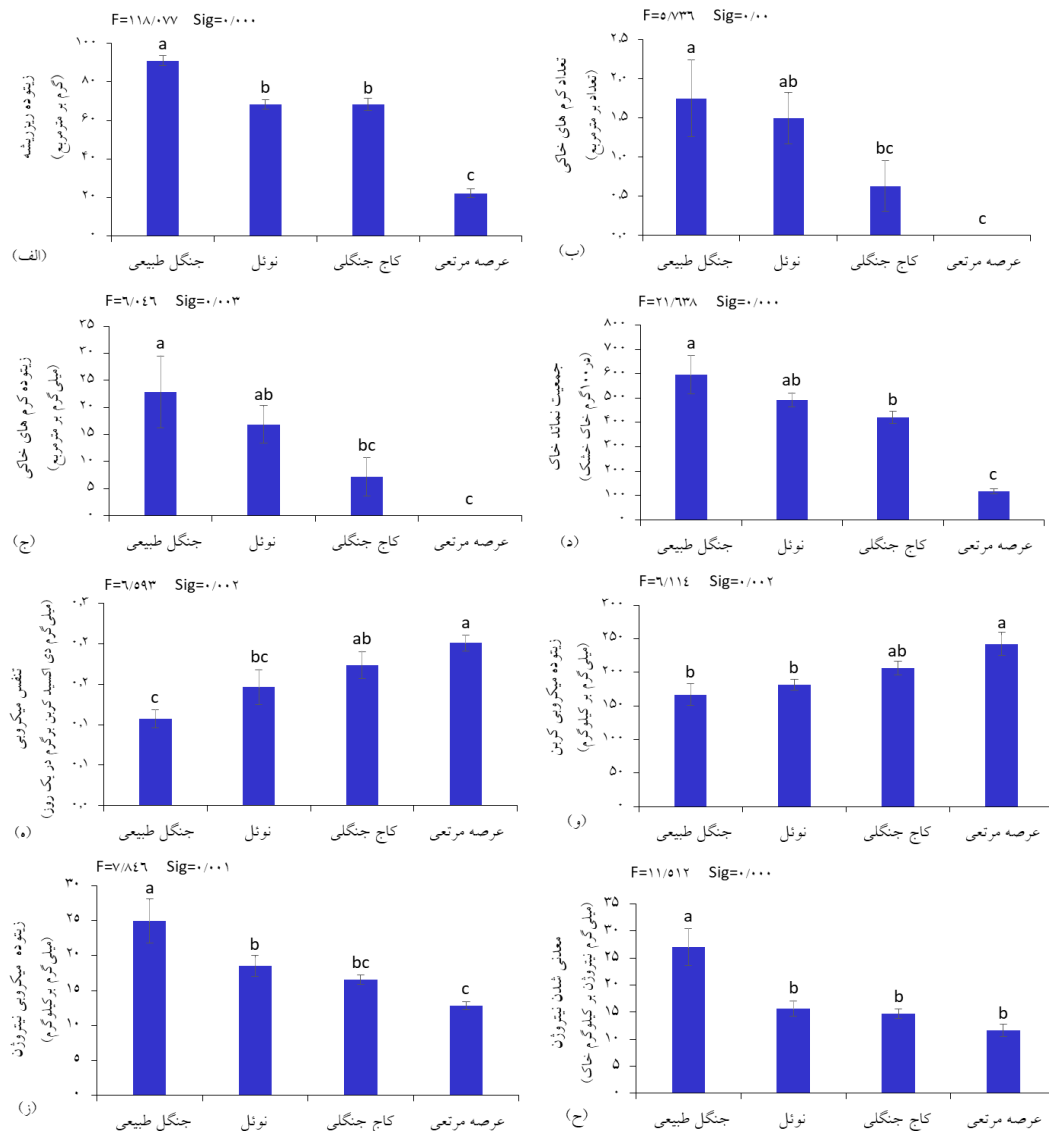
شکل ۲- میانگین (±اشتباه معیار) فعالیت‌های زیستی خاک در کاربری‌های مختلف Figure 2. Mean (±SE) of soil biological activities in different land uses
