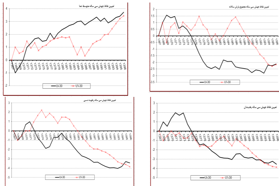
شکل ۸- نمودار آزمون من-کندال برای بارش، دما، رطوبت نسبی و یخبندان بازه زمانی ۳۰ سال در منطقه مورد مطالعه
