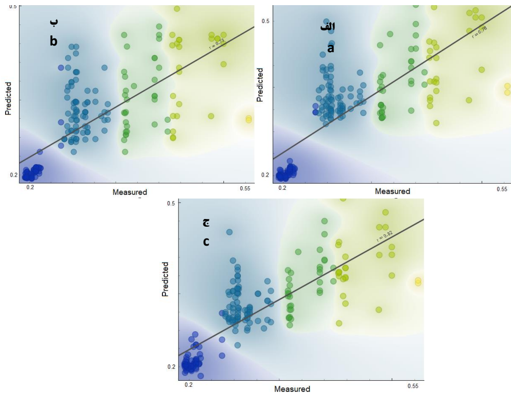
شکل ۶- ارزیابی دقت روش های مختلف، درخت تصمیم (الف)، جنگل تصادفی (ب) و تقویت گرادیان (ج) Figure 6. Accuracy evaluation of different methods; decision tree (a), random forest (b) and gradient boosting (c)
