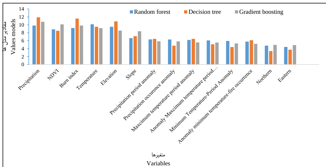
شکل ۷- اهمیت پارامترهای مختلف در سه مدل مورد بررسی Figure 7. The importance of different parameters in the three investigated models
