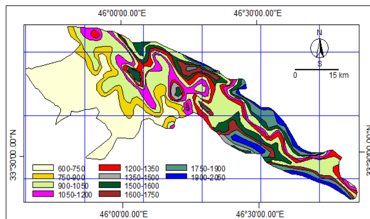
شکل ۲- طبقات ارتفاعی منطقه مورد مطالعه Figura 2. Elevation classes in the study area
