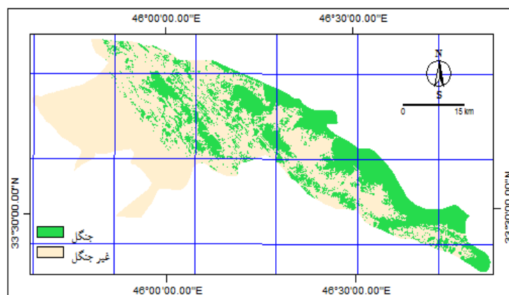
شکل ۴- گستره جنگل و غیرجنگل سال ۱۳۸۰ حاصل از پردازش تصاویر ماهواره‌ای لندست هفت سنجنده ETM + Figura 4. Cobertura forestal y no forestal en 2001, como resultado del procesamiento de Satellite imagery processing Landsat 7 ETM +
