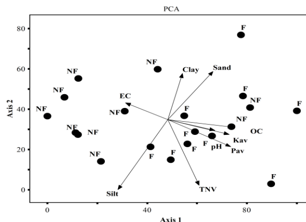
شکل ۵- رج‌بندی خصوصیات فیزیکی و شیمیایی خاک مورد بررسی در فضای دو مؤلفه اول و دوم (EC: هدایت الکتریکی، Clay: درصد رس، Sand: درصد شن، OC: کربن آلی، Kav: پتاسیم در دسترس، Pav: فسفر در دسترس، pH: اسیدیته، TNV: آهک و Silt: درصد سیلت)
