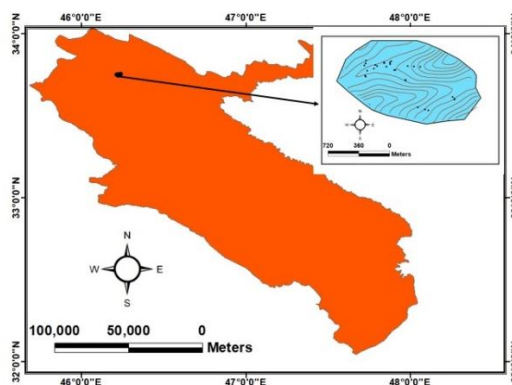
شکل ۱- موقعیت منطقه مورد پژوهش در نقشه استان ایلام
