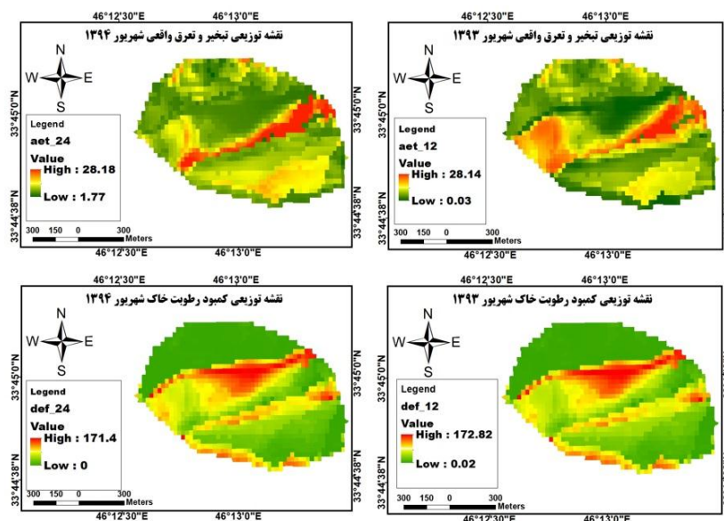
شکل ۲- نقشه‌های توزیعی مولفه‌های بیلان در رویشگاه جنگلی مله‌سیاه ایلام
