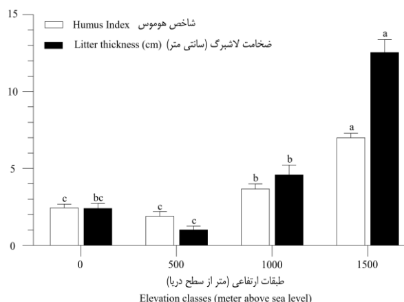
شکل ۲- مقایسه شاخص هوموس و ضخامت لاشبرگ در طبقات مختلف ارتفاعی Figure 2. Comparison of humus index and litter thickness in different elevation classes
