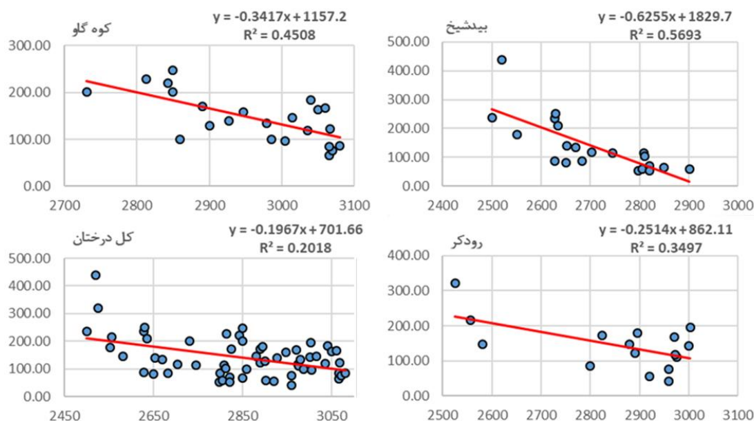
شکل ۳- معادله خط رگرسیون متغیر ارتفاع از سطح دریا (محور X) و متغیر متوسط پهنای حلقه رویشی (محور Y) Figure 3. Linear regression equation for altitude (x-axis) and average ring width growth (y-axis)
