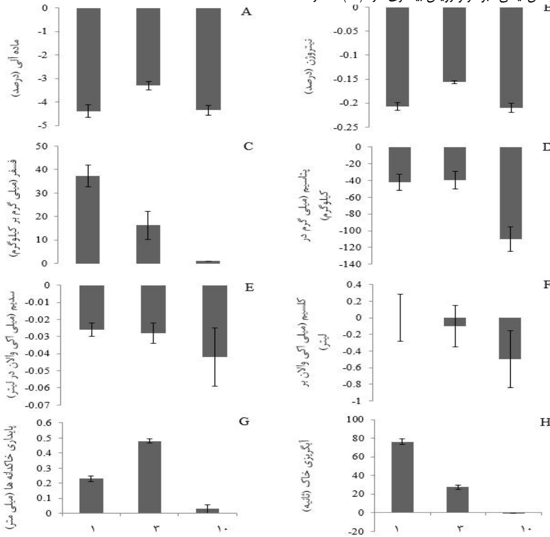
شکل ۱- میزان کاهش یا افزایش عناصر غذایی و پایداری خاکدانه‌ها در سال‌های پس از آتش‌سوزی: کربن آلی (A)، نیتروژن (B)، فسفر (C)، پتاسیم (D)، سدیم (E)، کلسیم (F)، پایداری خاکدانه‌ها (G)، آبگریزی خاک (H)
