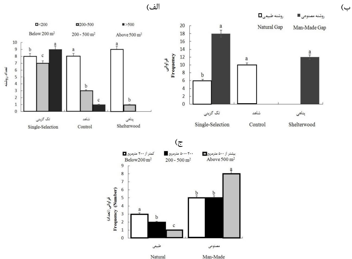
شکل ۴- فراوانی سطح روشن‌ها (الف)، فراوانی انواع روشن‌ها در قطعات تک‌گزینی، شاهد و تدریجی-پناهی (ب) و مقایسه فراوانی سطح روشن‌های طبیعی و مصنوعی در قطعه تک‌گزینی (ج)
