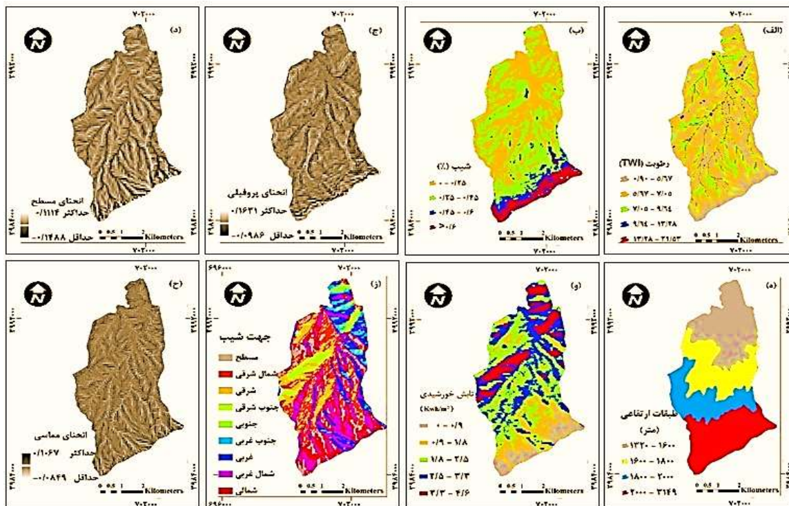
شکل ۲- نقشه خصوصیات اولیه و ثانویه توپوگرافی- الف) شاخص رطوبت ب) شیب ج) انحنای پروفیلی د) انحنای مسطح ه) طبقات ارتفاعی و) تابش خورشیدی ز) جهت شیب ح) انحنای مماسی Figure 2. Map of primary and secondary features of topography- A) Wetness Index B) Slope C) Profile C. D) Plan C. E) Elevation F) Solar Radiation G) Aspect H) Tangential C.
