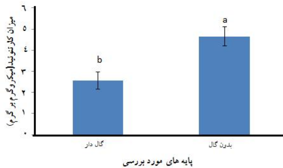
شکل ۸- میزان کاروتنوئید (میکروگرم بر گرم) در سرشاخه‌های بدون گال و گال‌دار درختان بلوط ایرانی Figure 8. Carotenoids (µg/g) in twigs with and without gall in Iranian oak trees
